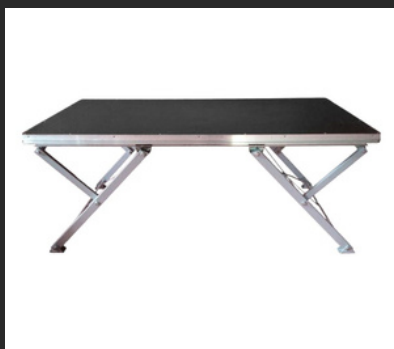
ESTRADO TESOURA GUIL
